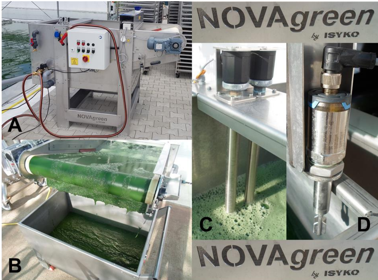
Abbildung 6: Überarbeitetes Modell des Bandfiltererntegerätes der Firma NOVAgreen Projektmanagement GmbH (A, B). Füllstandsensoren zur Messung bzw. Steuerung von Zulauf und Produkt (C, D).
